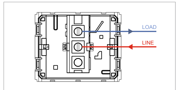
Wiring Diagram:
